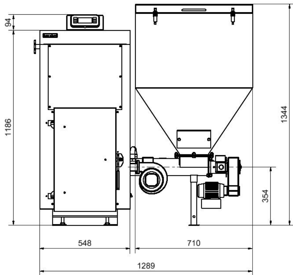
Obr. č. 3 Základní rozměry kotle BENEKOV C17 (verze PREMIUM)
