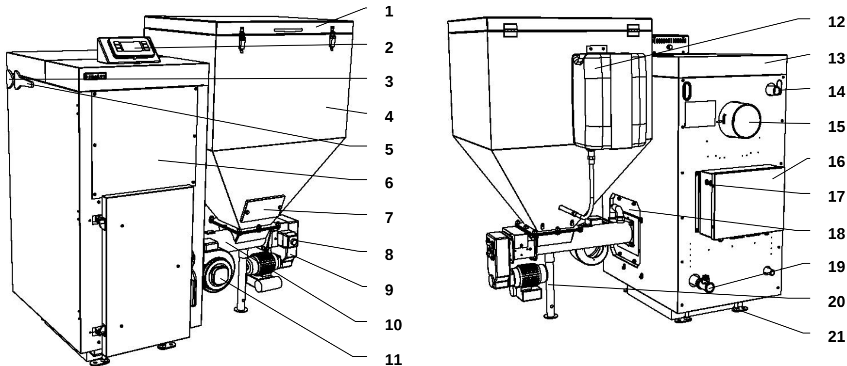
Obr. č. 1 Čelní a zadní pohled kotlů BENEKOV C17 a C27 (verze PREMIUM)
