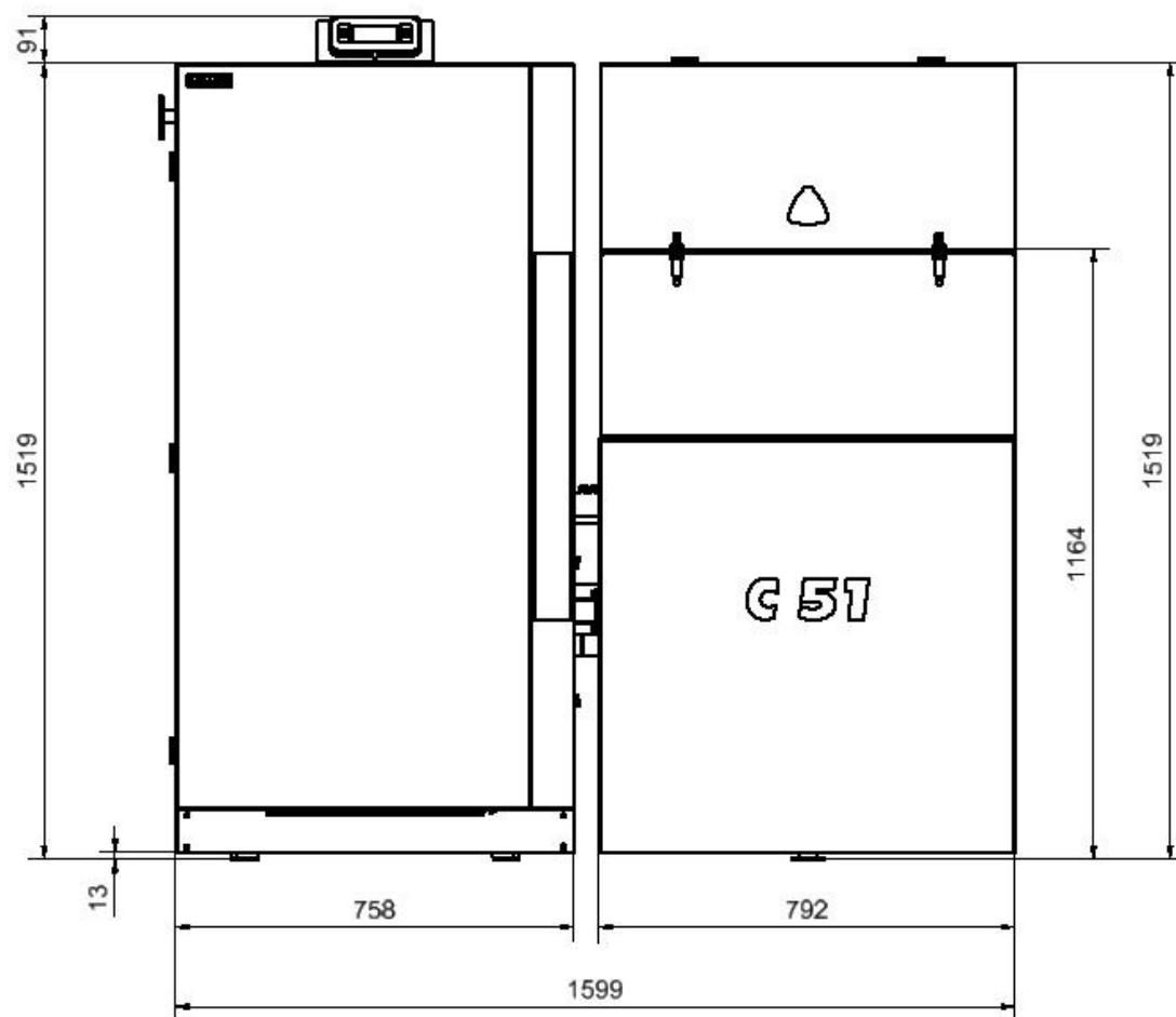
Obr. č. 6 Základní rozměry kotle BENEKOV C51
