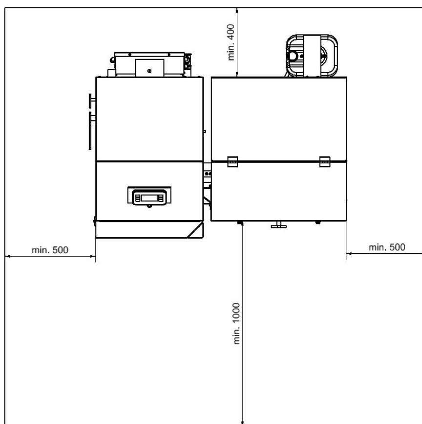
Obr. č. 7 Umístění kotle v kotelně
