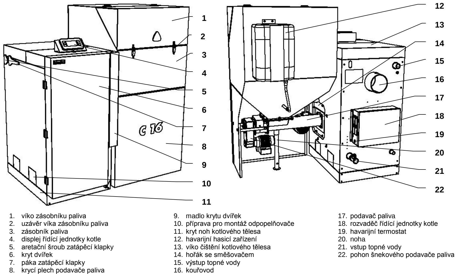
Obr. č. 1 Čelní a zadní pohled kotle BENEKOV C16
