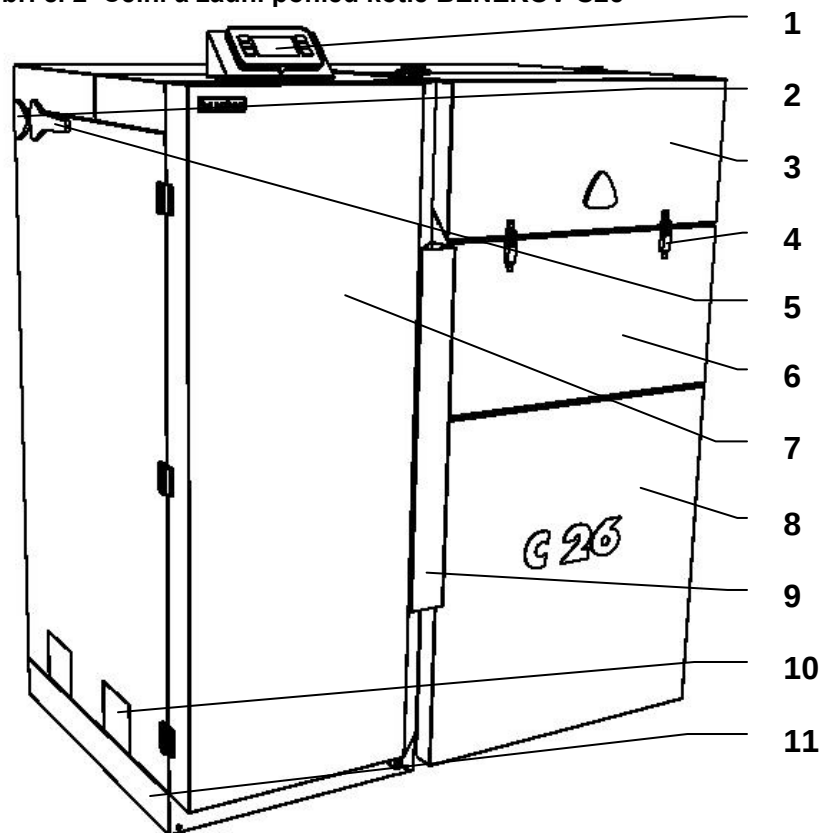
Obr. č. 2 Čelní a zadní pohled kotle BENEKOV C26
