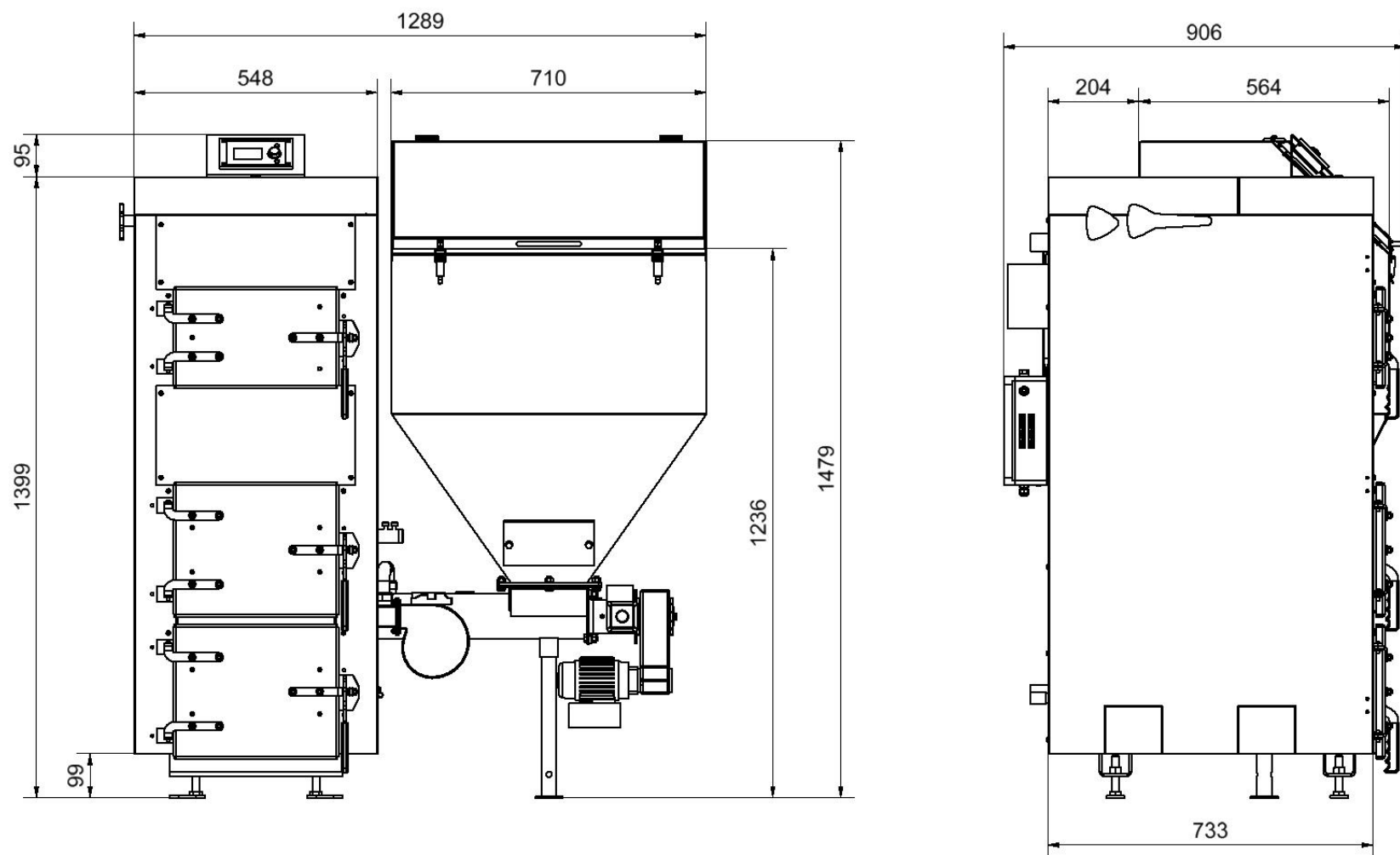
Obr. č. 2 Základní rozměry kotle CosmoTHERM U26
