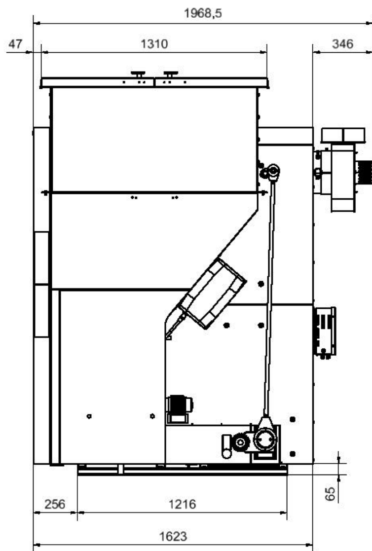
Obr. č. 3 Základní rozměry kotle BENEKOV R100 (s přídatným modulem zásobníku paliva)
