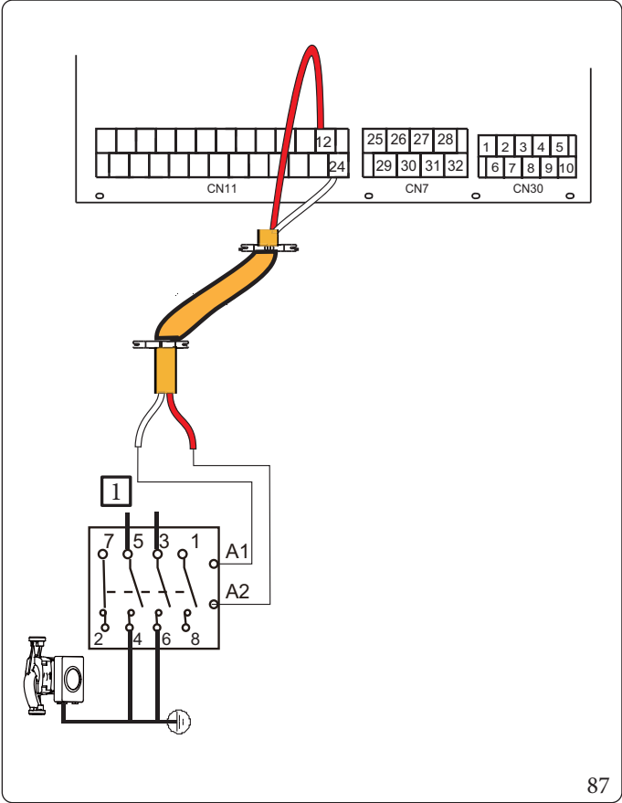
Vysvětlivky (obr. 87): 1 - Napájení
