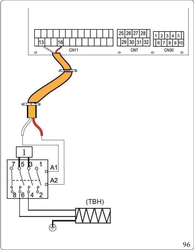
Vysvětlivky (Obr. 96): 1 - Napájení
