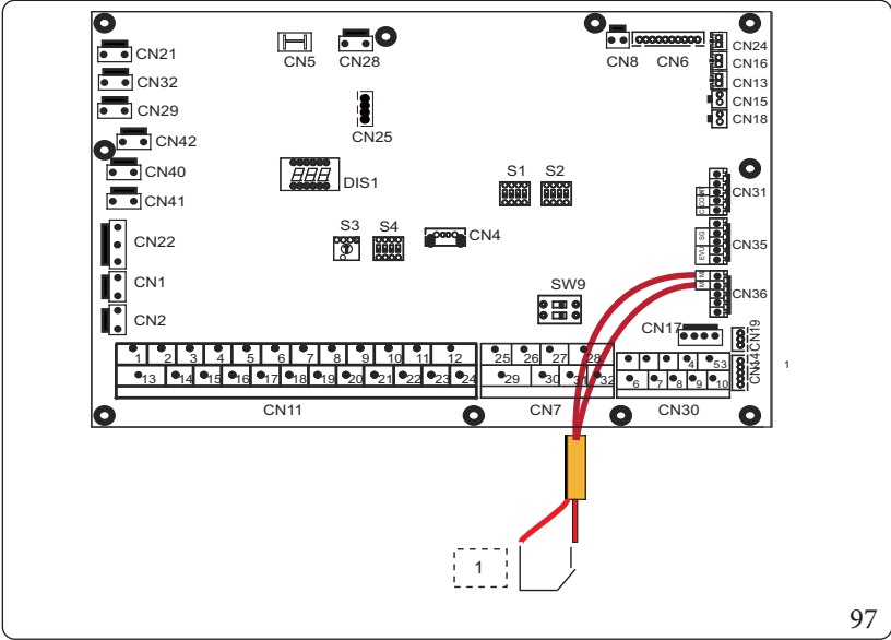
Vysvětlivky (Obr. 97): 1 - Zavřete: Vypnutí
