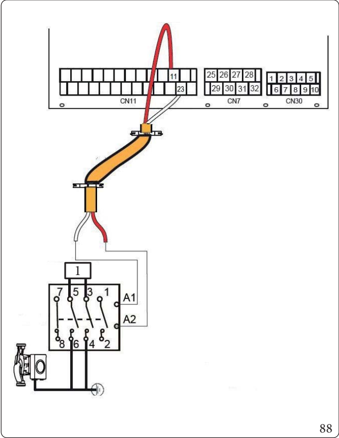
Vysvětlivky (obr. 88): 1 - Napájení
