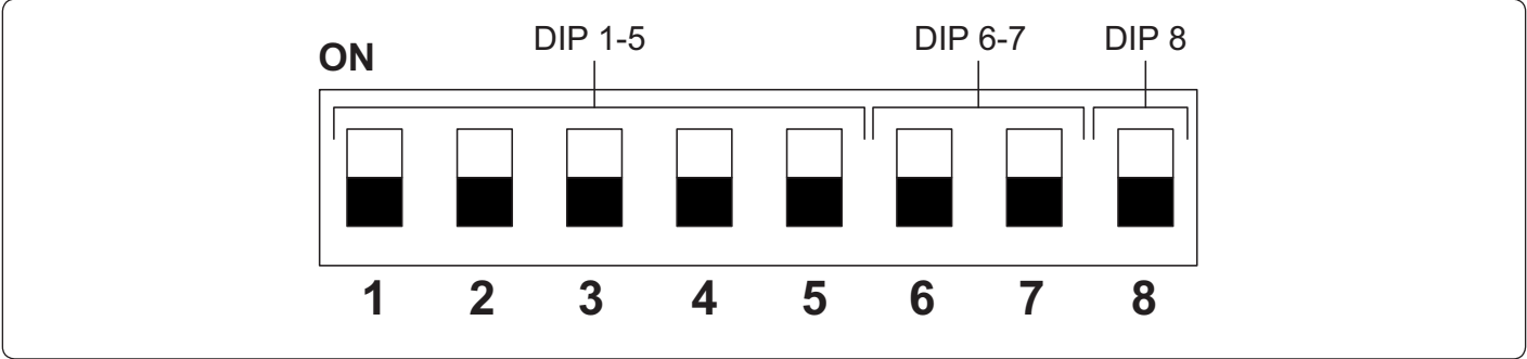
Konfigurační tabulka spínače DIP-Switch
