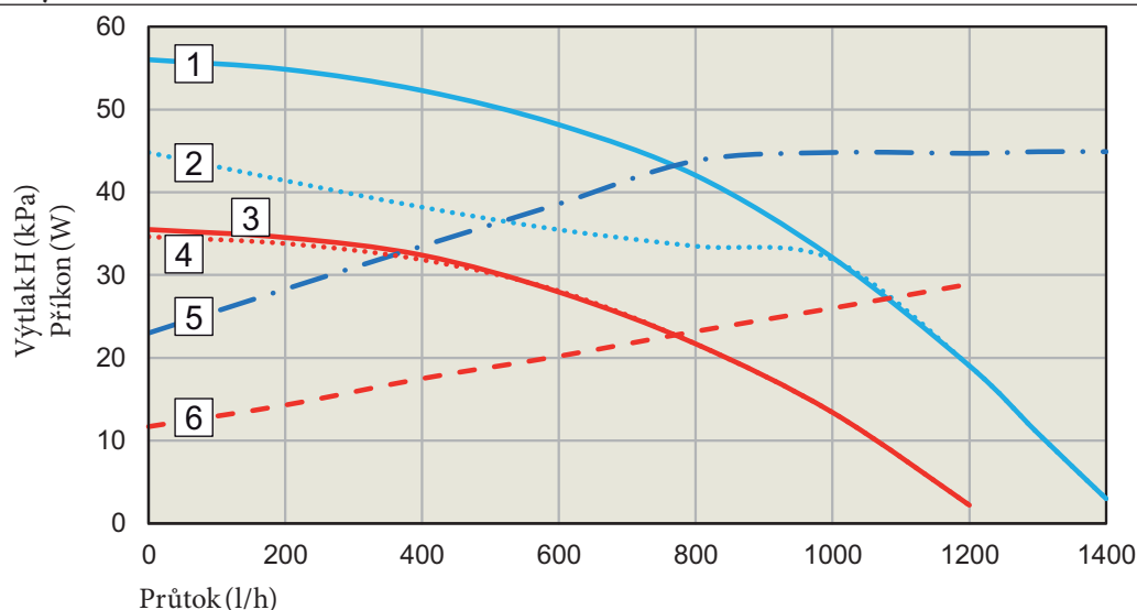
Graf průtoku - Výtlak - Příkon VICTRIX TERA V3 24 PLUSEU
