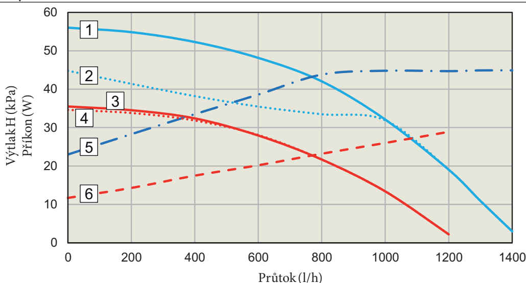
Graf průtoku - Výtlak - Příkon VICTRIX TERA V3 28 E
