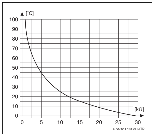
Obr. 11 Charakteristika odporu čidla teploty (vyjma venkovní teploty)
