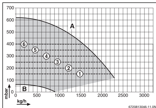
Obr. 10 Zbytková dopravní výška u GC9000iW 50
