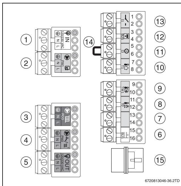
Obr. 27 Svorkovnice
