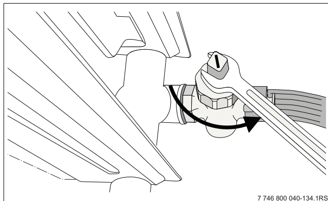
Obr. 41 Vypuštění topného systému při nebezpečí mrazu
