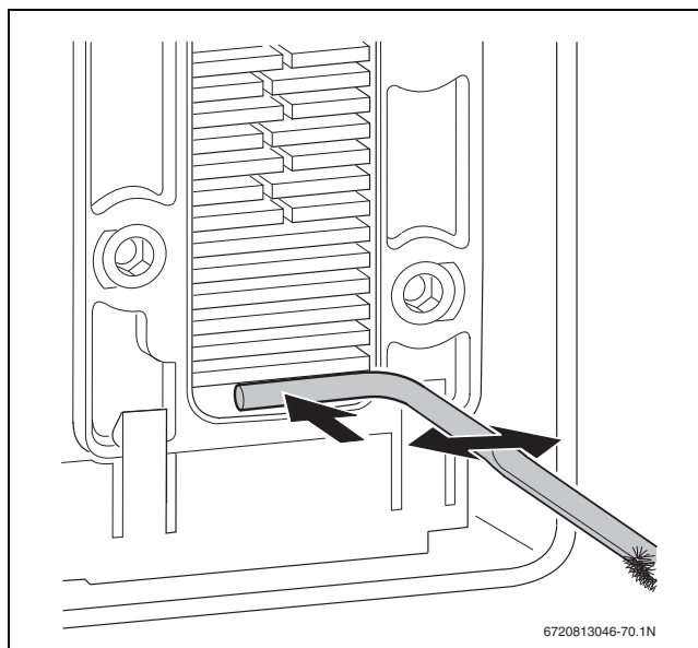
Obr. 52 Čištění vany kondenzátu
