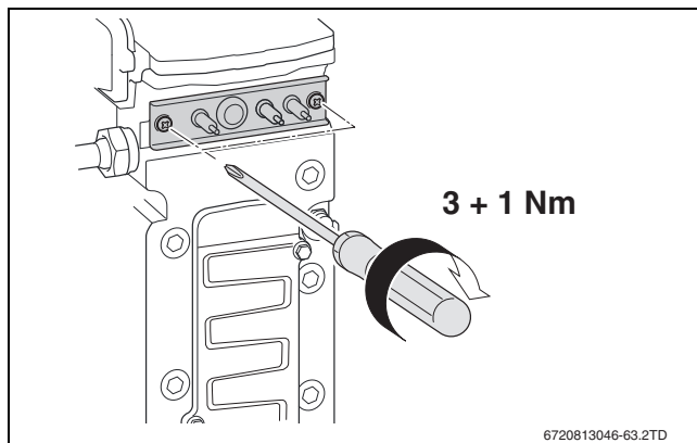
Obr. 42 Montáž sady elektrod
