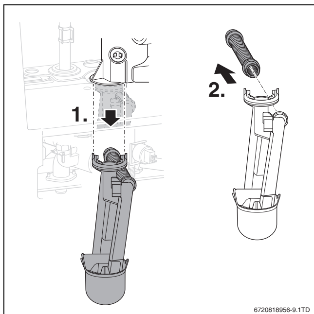
Obr. 47 Sifon kondenzátu
