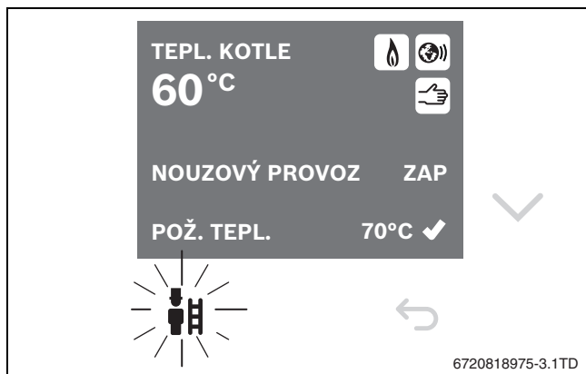
Obr. 38 Menu Nouzový provoz
