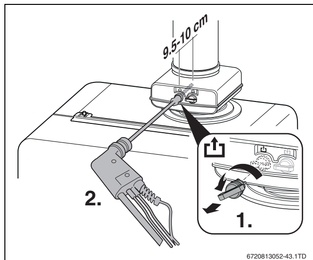
Obr. 32 Měření obsahu CO/CO 2
