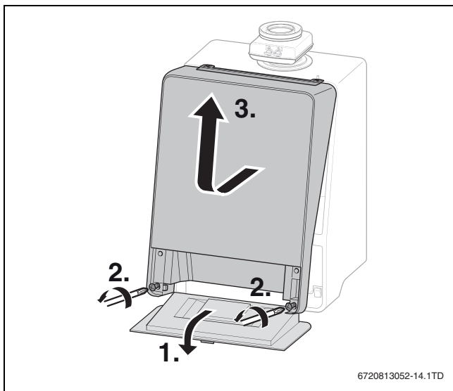
Obr. 18 Demontáž opláštění zařízení
