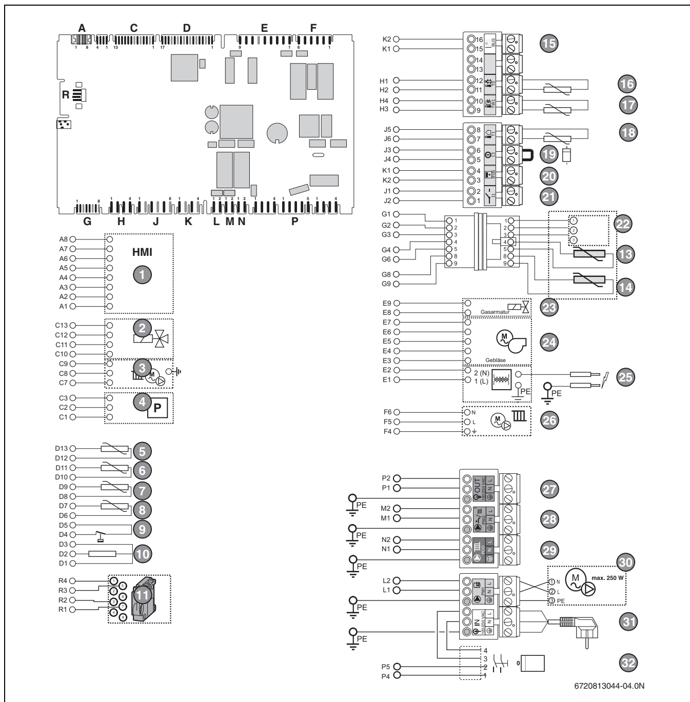
Obr. 6 Řídicí deska
