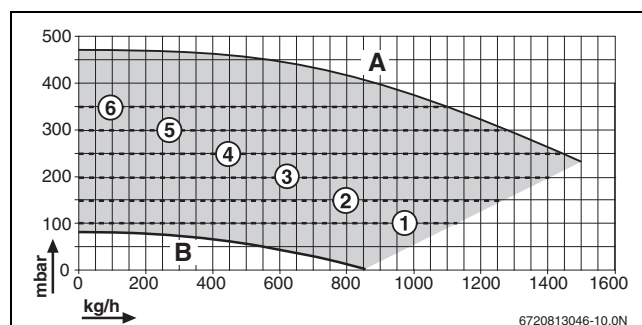
Obr. 9 Zbytková dopravní výška u GC9000iW 40
