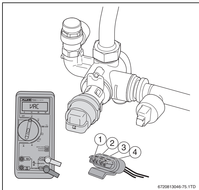
Obr. 53 3cestný ventil
