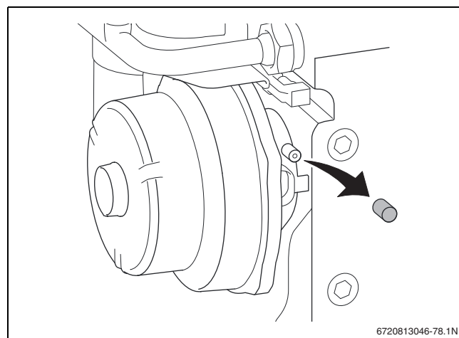
Obr. 48 Měřicí hrdlo na směšovacím zařízení
