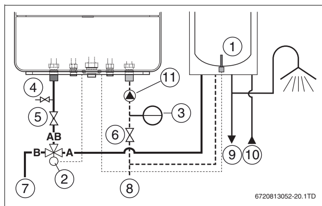
Obr. 22 Montáž externího 3cestného ventilu (230 V)
