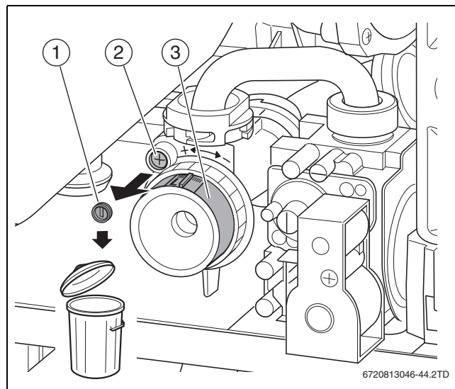
Obr. 31 Odstranění plomby
