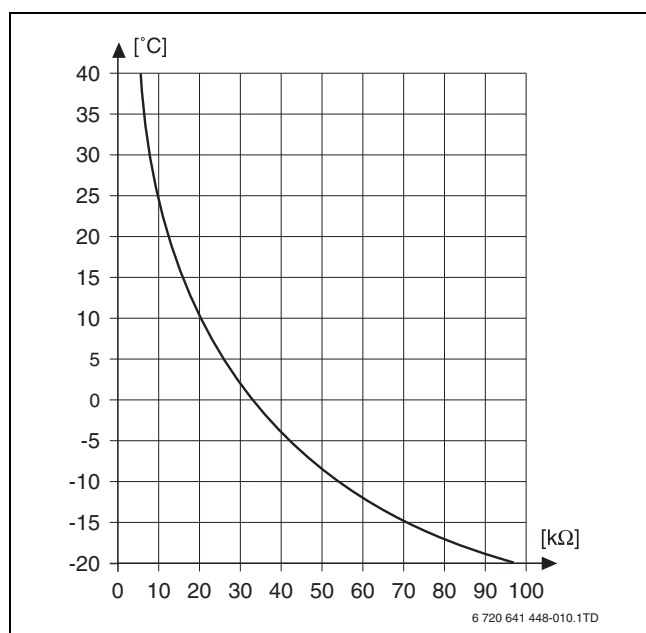
Obr. 12 Charakteristika odporu pro čidla venkovní teploty
