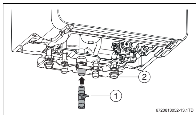
Obr. 17 Připojení plynu
