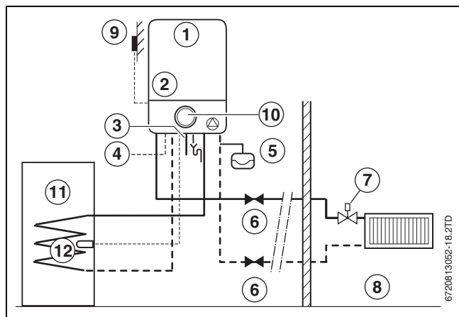
Obr. 21 Příklad aplikace s regulací podle venkovní teploty a zásobníkem teplé vody
