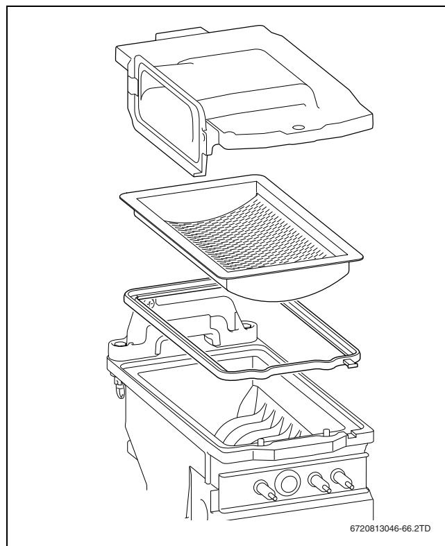
Obr. 45 Vyjmutí hořáku
