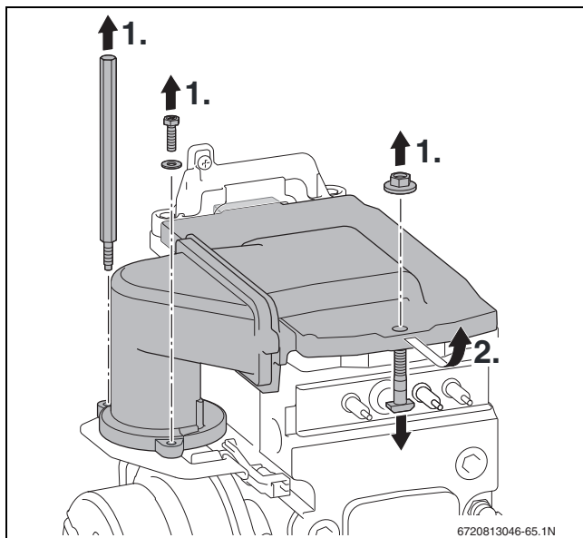
Obr. 44 Odmontování horního krytu hořáku
