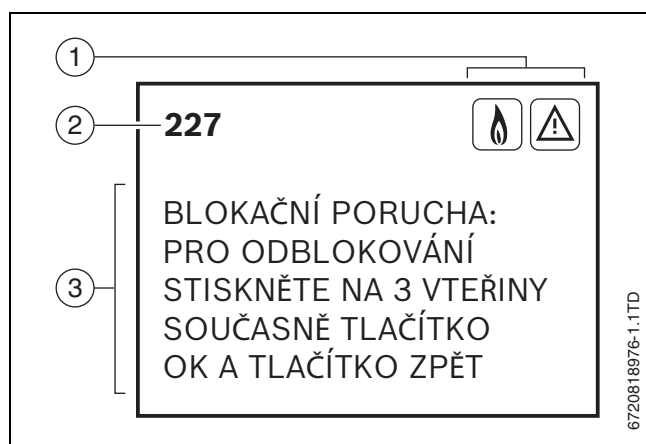
Obr. 54 Menu poruch
