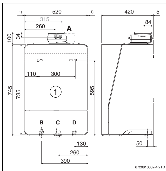
Obr. 5 Rozměry a přípojky [mm]
