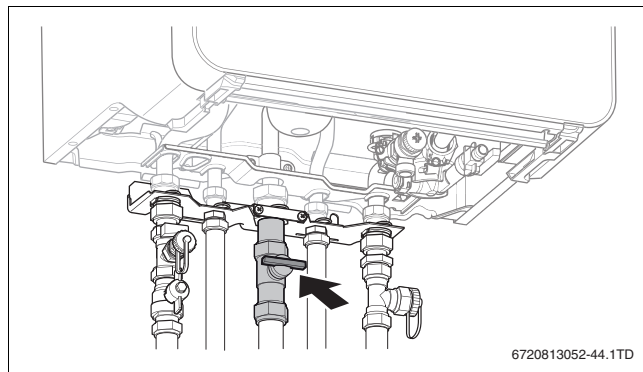
Obr. 40 Plynový ventil zavřený
