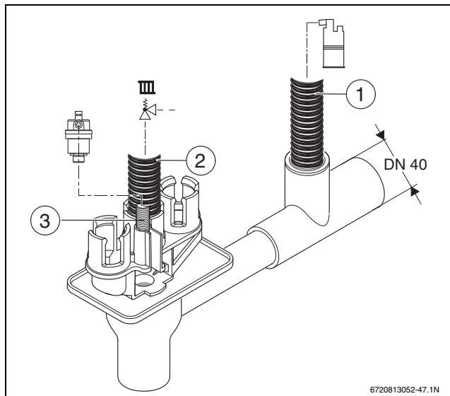
Obr. 23 Montáž hadice kondenzátu a hadice od pojistného ventilu a odvzdušňovače
