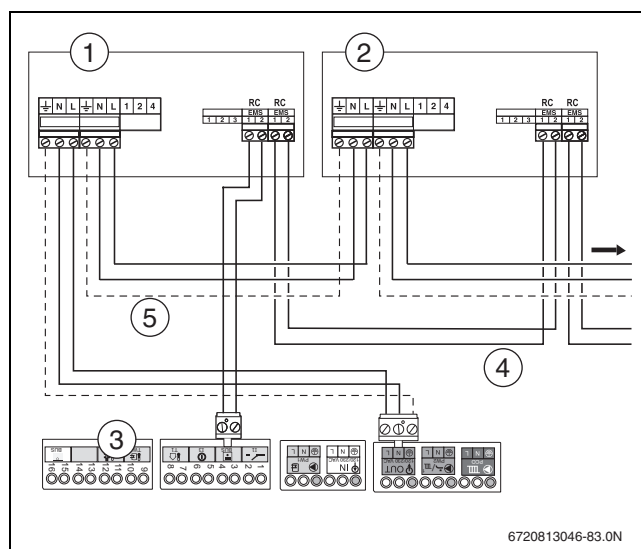
Obr. 28 Připojení několika modulů
