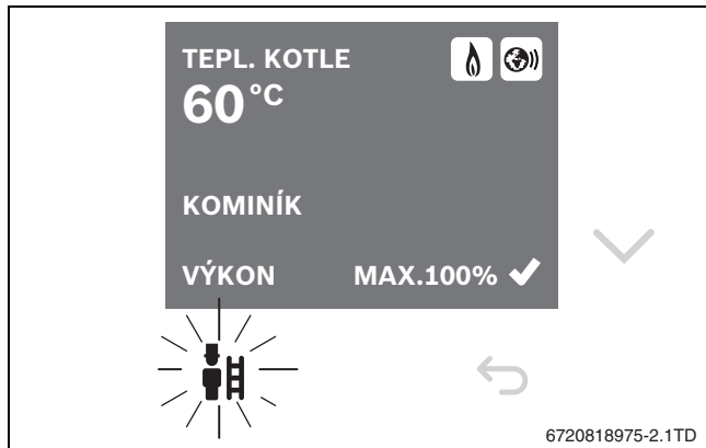
Obr. 37 Menu pro kominický provoz
