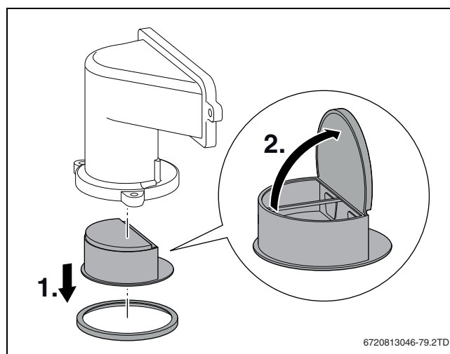
Obr. 46 Zpětná klapka ve směšovacím zařízení
