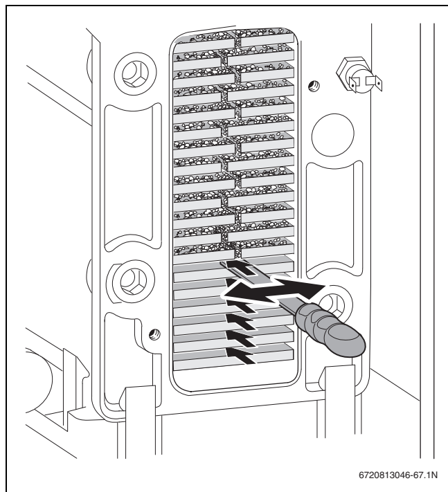
Obr. 49 Čisticí nůž
