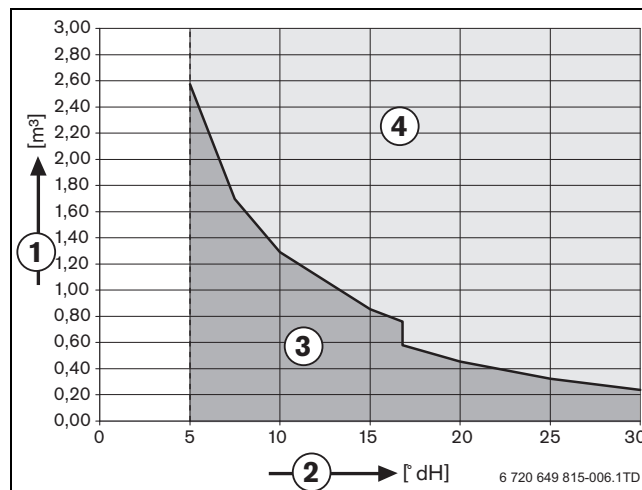
Obr. 14 Požadavky na plnicí a doplňovací vodu u přístrojů < 50 kW
