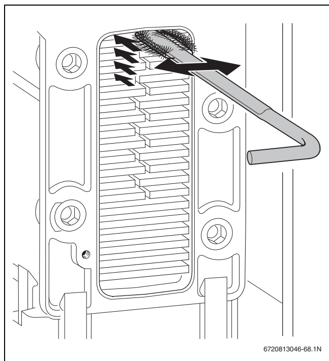
Obr. 50 Čištění tepelného bloku kartáčem
