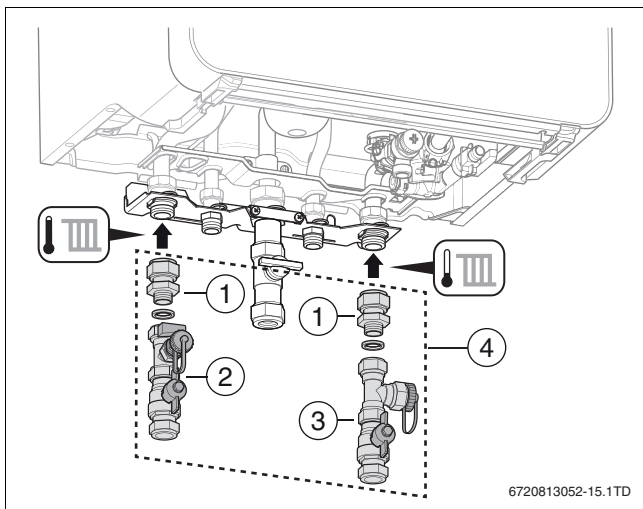
Obr. 19 Připojení potrubí otopné vody na zařízení
