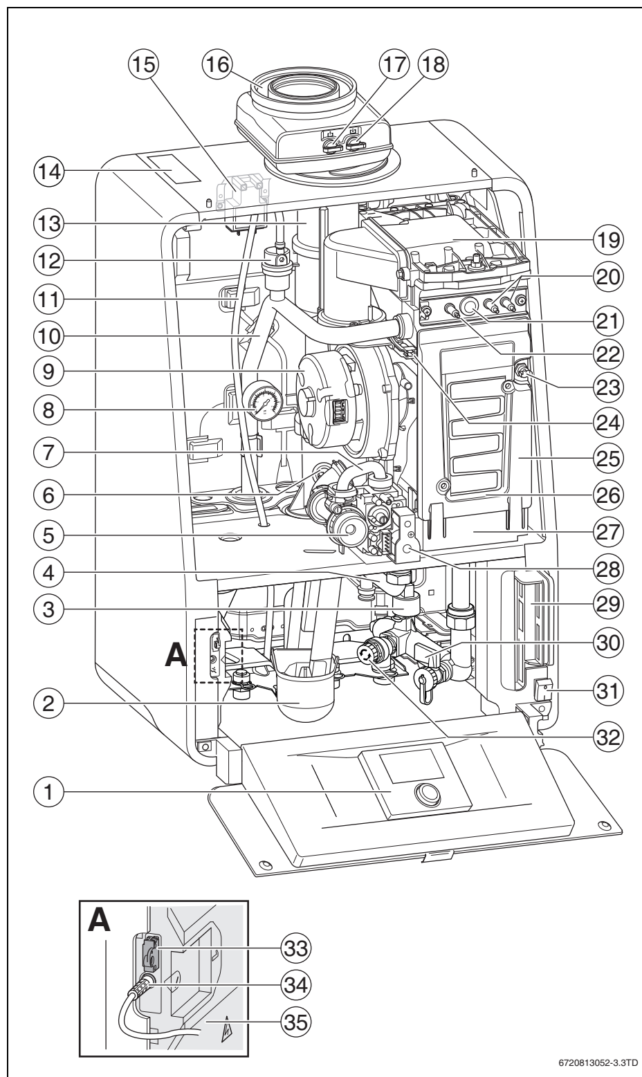
Obr. 3 GC9000iW 40/50
