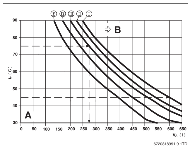
Obr. 20 Charakteristiky expanzní nádoby, expanzní nádoba vytápění o obsahu 14 l
