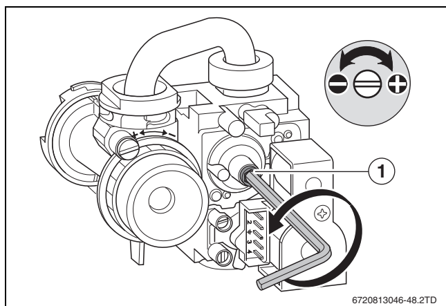
Obr. 33 Odstranění plomby
