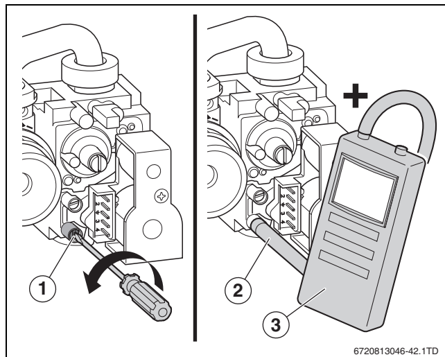
Obr. 30 Měření přípojovacího přetlaku plynu
