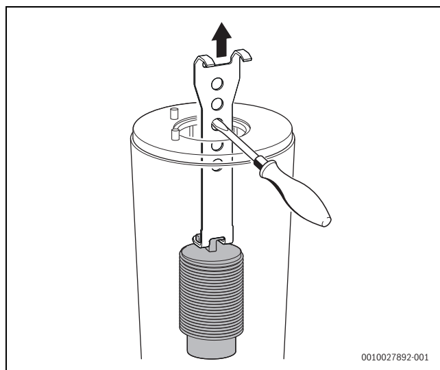
Obr. 171 Vyjmutí spodního výtlačného tělesa
