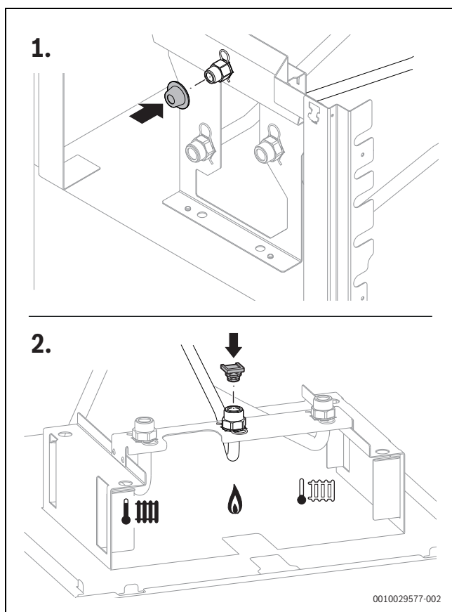
Obr. 58 Nasazení krytky a zásepky na plynové potrubí
