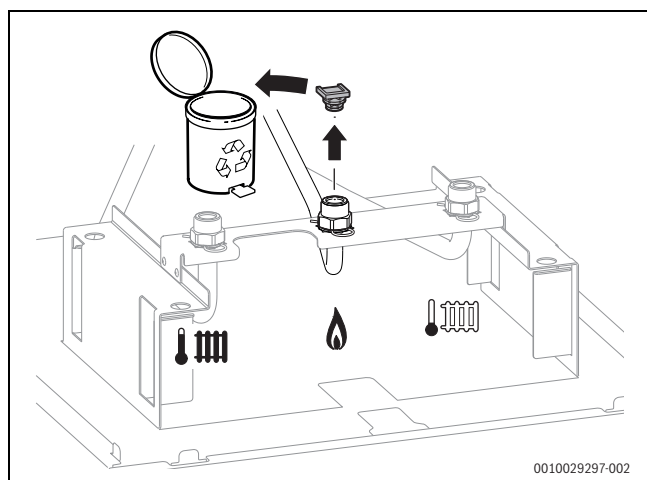
Obr. 68 Odstranění zásepek na plynovém potrubí
