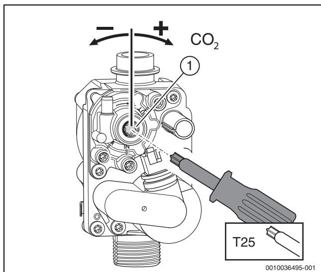
Obr. 156 Nastavení obsahu \text{CO}_2/\text{O}_2 při minimálním jmenovitém tepelném výkonu
