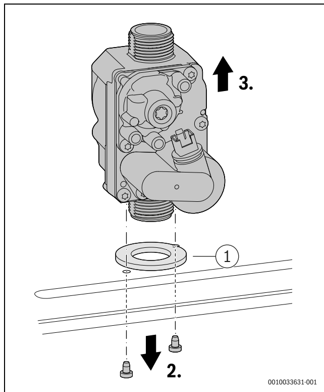
Obr. 187 Demontáž plynového ventilu
