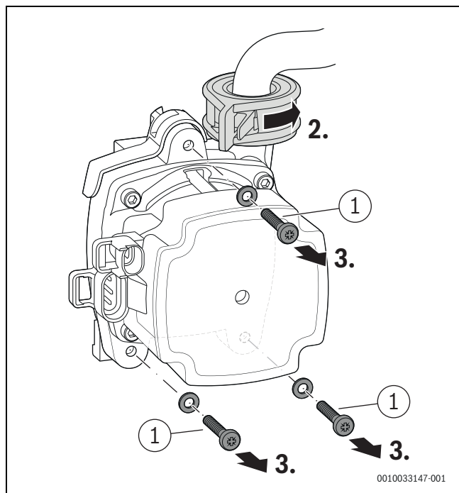
Obr. 181 Odjistění čerpadla otopného systému a odstranění šroubů
