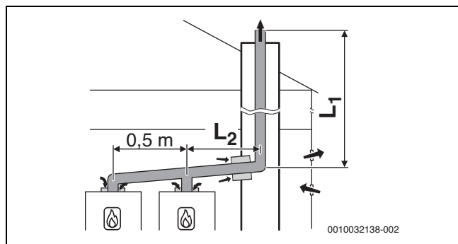
Obr. 43 Kaskáda se 2 zařízeními: Pevné vedení odvodu spalin v šachtě podle B 23p /B 53p s přívodem vzduchu závislým na vzduchu z prostoru na zařízení
