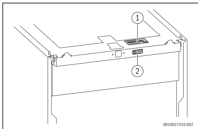
Obr. 3 Umístění typových štítků
