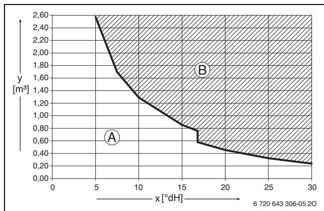
Obr. 45 Požadavky na plnicí a doplňovací vodu v °dH u zařízení < 50 kW
