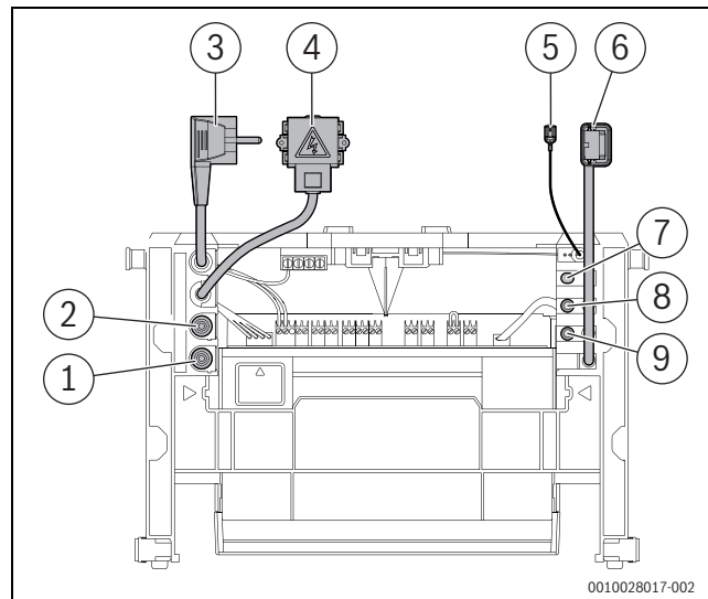
Obr. 132 Řídicí jednotka s připojenými součástmi ve stavu při dodání
