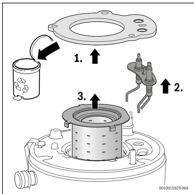
Obr. 169 Vymutí hořáku
