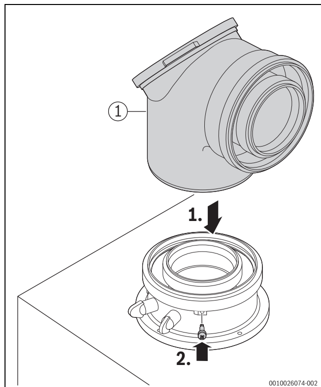
Obr. 77 Nasazení dílu systému odtahu spalin a zajištění šroubem
