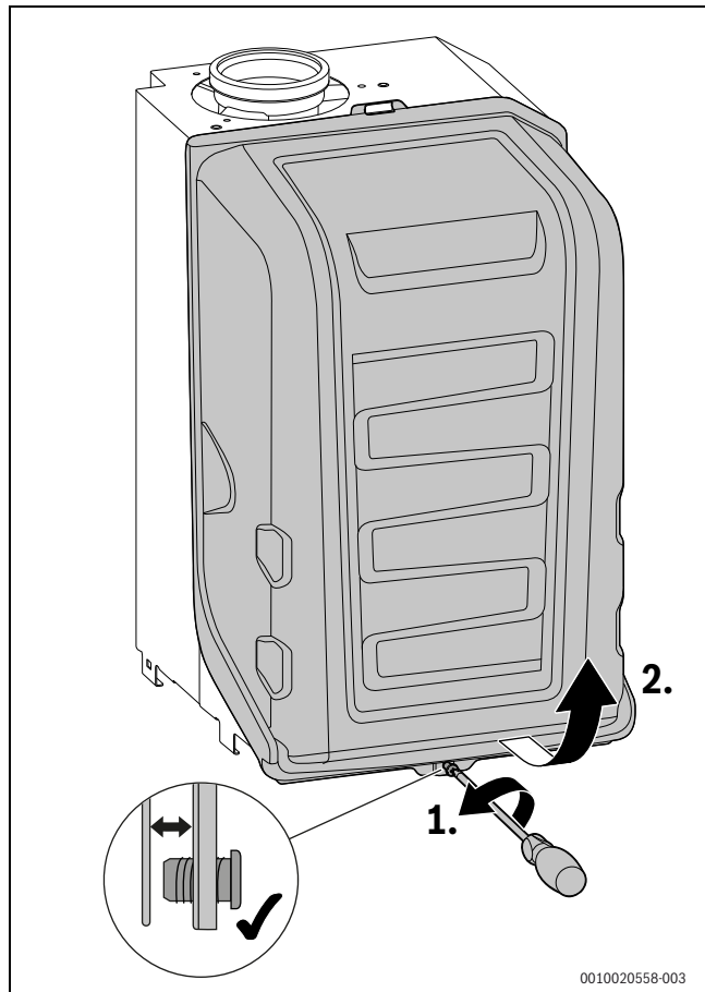
Obr. 153 Sejmутí krytu hořáku
