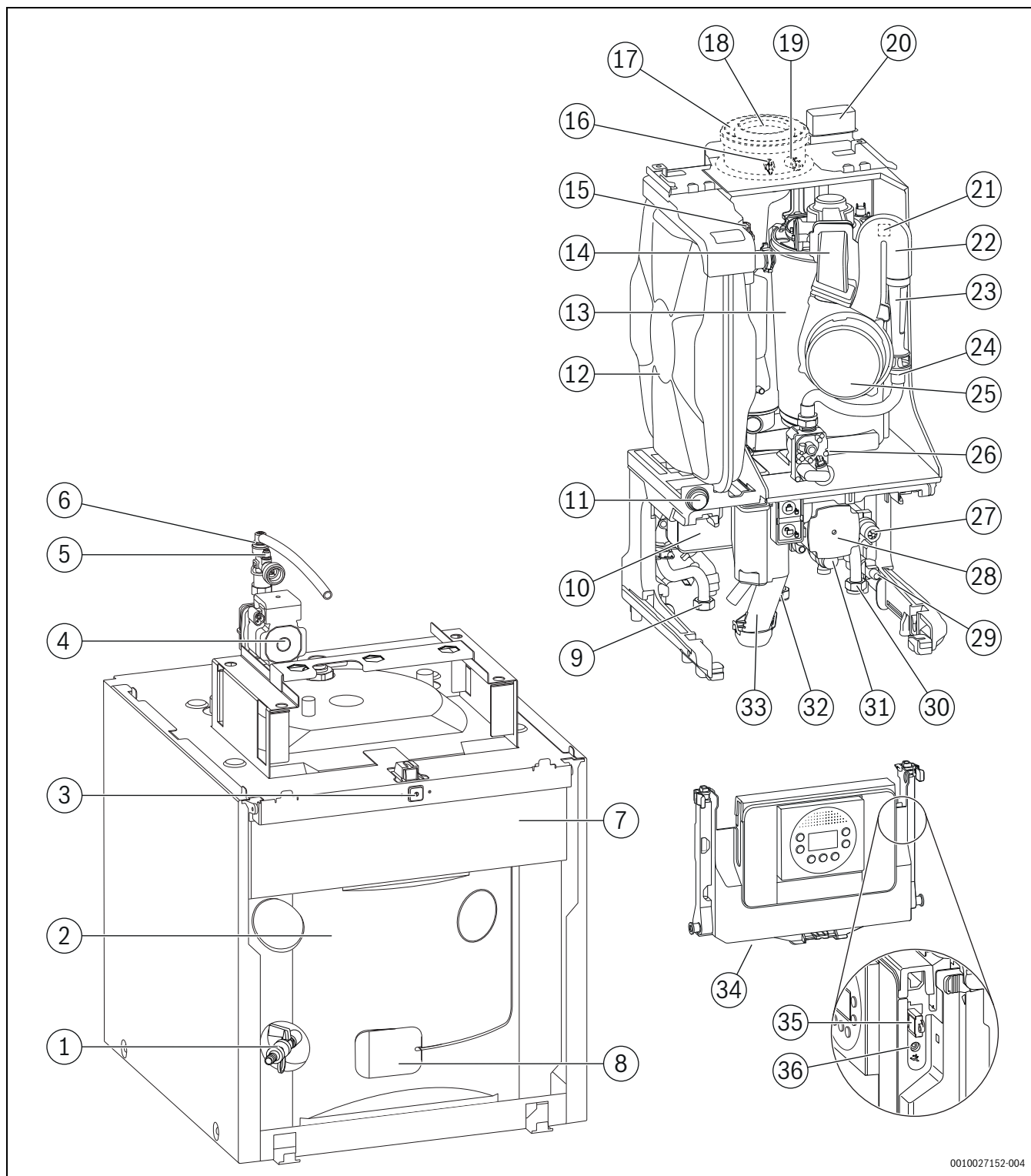
Obr. 5 Přehled výrobku
