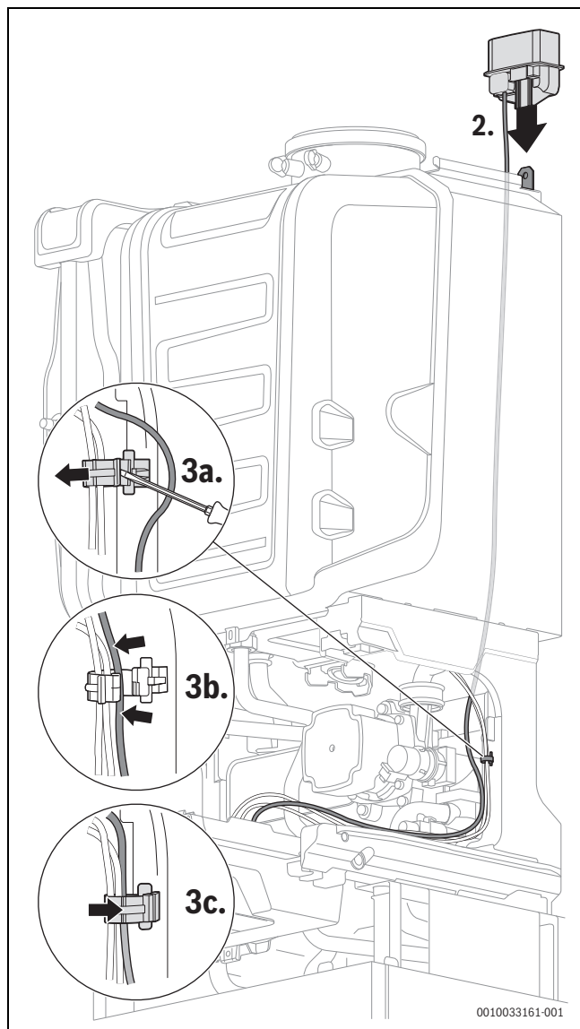
Obr. 75 Vsazení Key-slotu do konektoru pro přídatný modul a upevnění kabelu v kabelovém držáku
