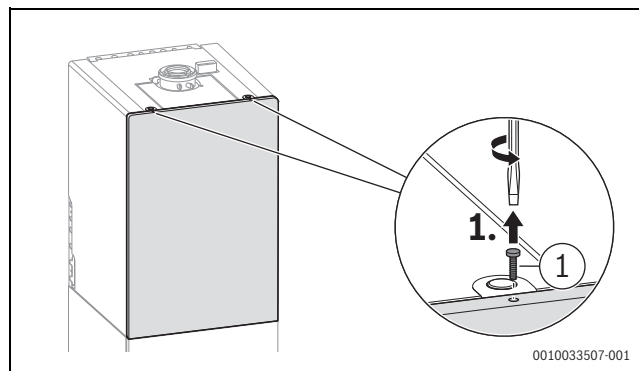
Obr. 157 Povolení zajišťovacího šroubu
