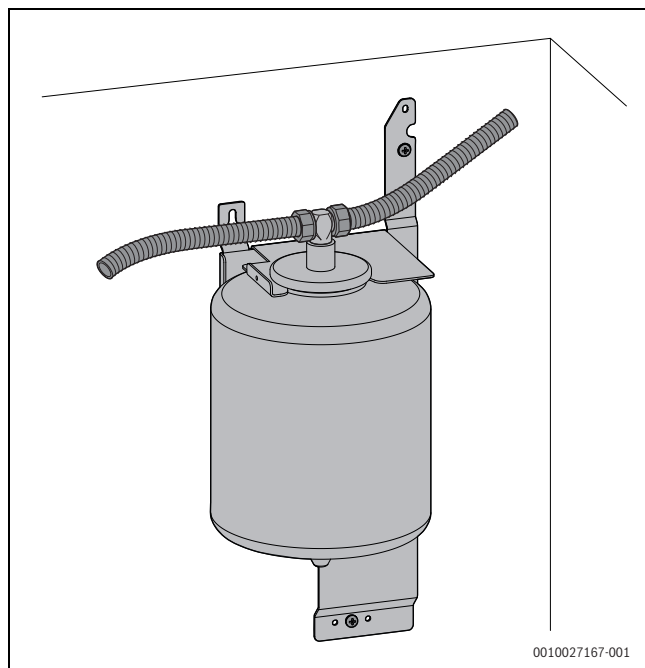
Obr. 108 Příslušenství EVW 8 namontované na stěnu
