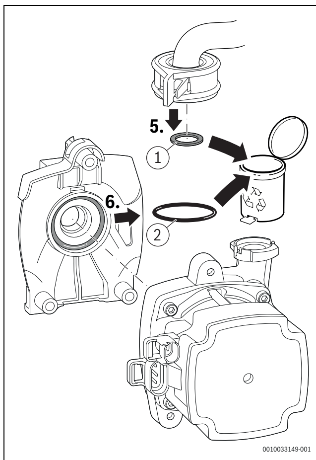
Obr. 183 Likvidace těsnění
