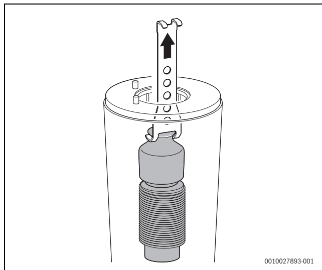
Obr. 170 Vyjmutí horního výtlačného tělesa
