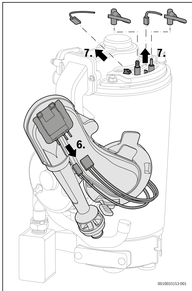
Obr. 165 Odpojení kabelů
