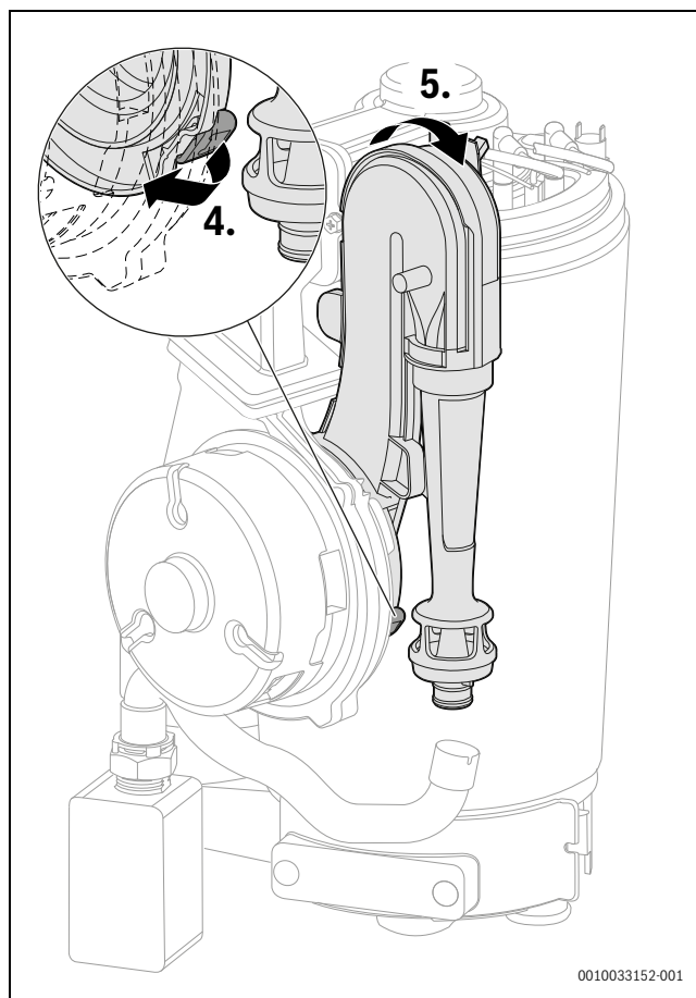
Obr. 164 Odebrání Venturiho trubice
