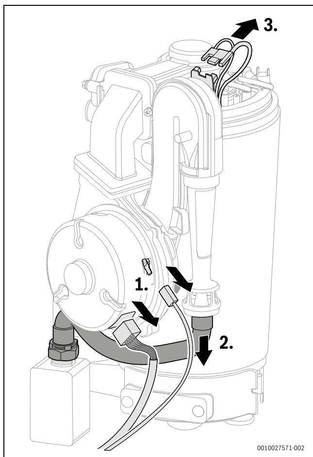
Obr. 163 Odpojení konektoru a plynové hadice
