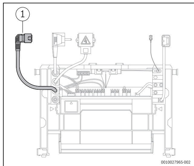
Obr. 133 Místo pro zasunutí připojovacího kabelu nabíjecího čerpadla stratifikačního zásobníku
