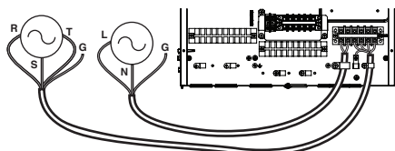
Záložní ohřivač 3Ø (Pro Hydrosplit)
