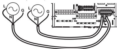
Záložní ohříváč 1Ø (Pro vnitřní jednotku Split R32 řady 4)
