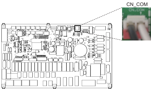
Vnitřní DPS
