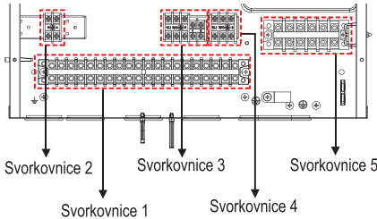
Pro 1Ø
