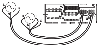
Záložní ohříváč 3Ø (Pro vnitřní jednotku Split R410A řady 3)
