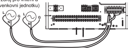
Záložní ohřivač 1Ø (Pro vnitřní jednotku Split R410A řady 5, Pro vnitřní jednotku Split R32 řady 5)
