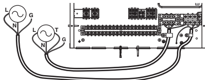
Záložní ohřivač 3Ø (Pro vnitřní jednotku Split R410A řady 5)
