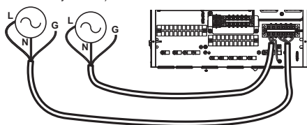
Záložní ohříváč 1Ø (Pro vnitřní jednotku Split R410A řady 3)
