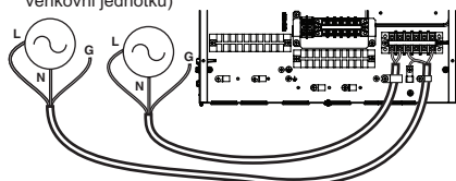
Záložní ohřivač 1Ø (Pro Hydrosplit)
