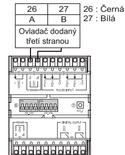
Rozhraní měřidla
