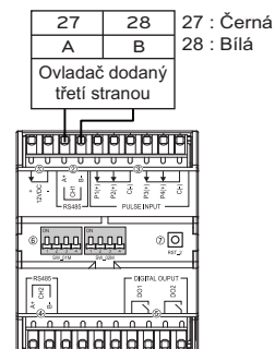
Rozhraní měřidla
