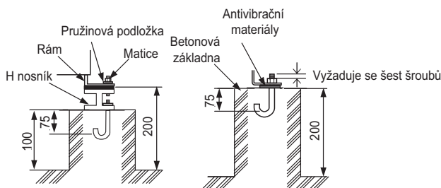
Způsob provedení základového šroubu
