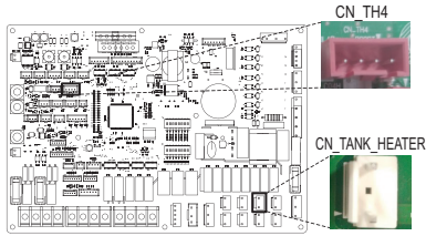
Vnitřní DPS
