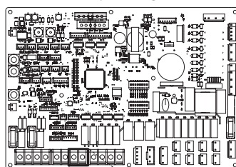
Vnitřní DPS
