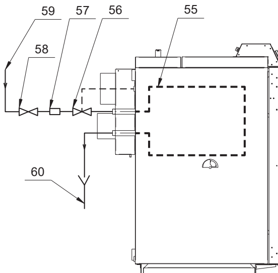
obr. 5 Připojení bezpečnostního ventilu ke kotli PYRO THERM
