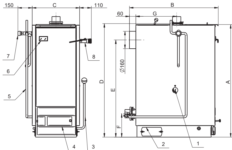
Obr. 1 Hlavní rozměry kotle SL27-4
