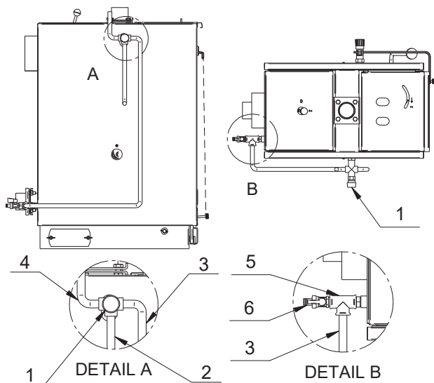
Obr. 7 Připojení DBV 1 ke kotlům VARIANT SL 27-4 a SL 33-4
