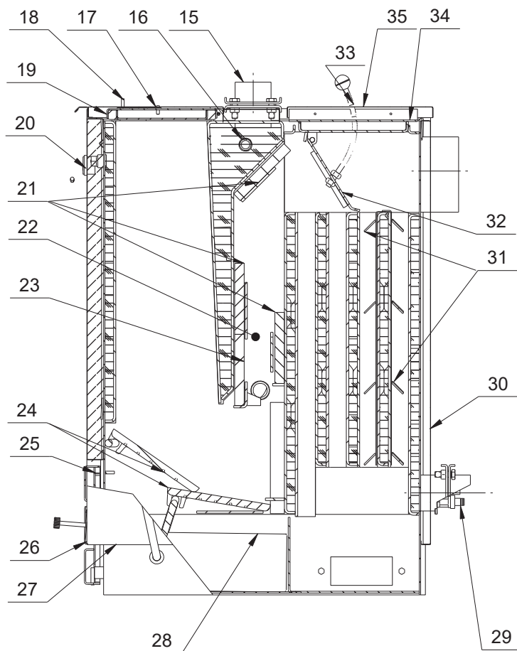
Obr. 2 Schéma kotle SL27-4
