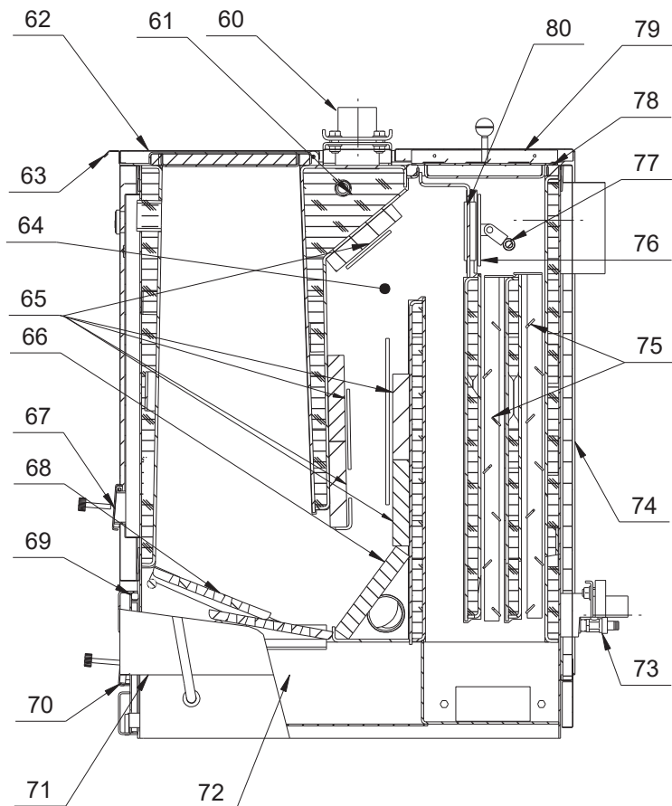
Obr. 4 Schéma kotle SL33-4
