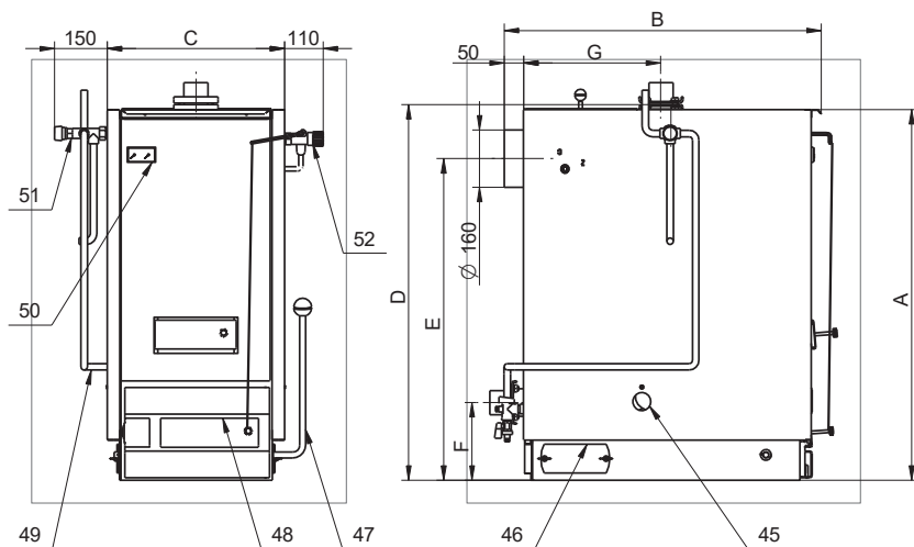
Obr. 3 Hlavní rozměry kotle SL33-4
