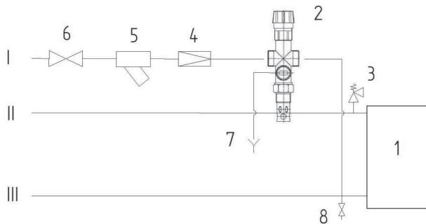
Obr. 8 Schéma zapojení DBV 1
